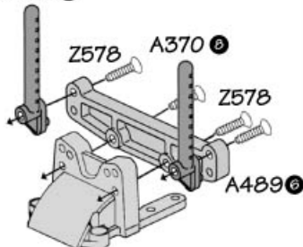
Z578 TP Flat H. Screw M3 x 12mm x 4 サラ タッピング ネジ
